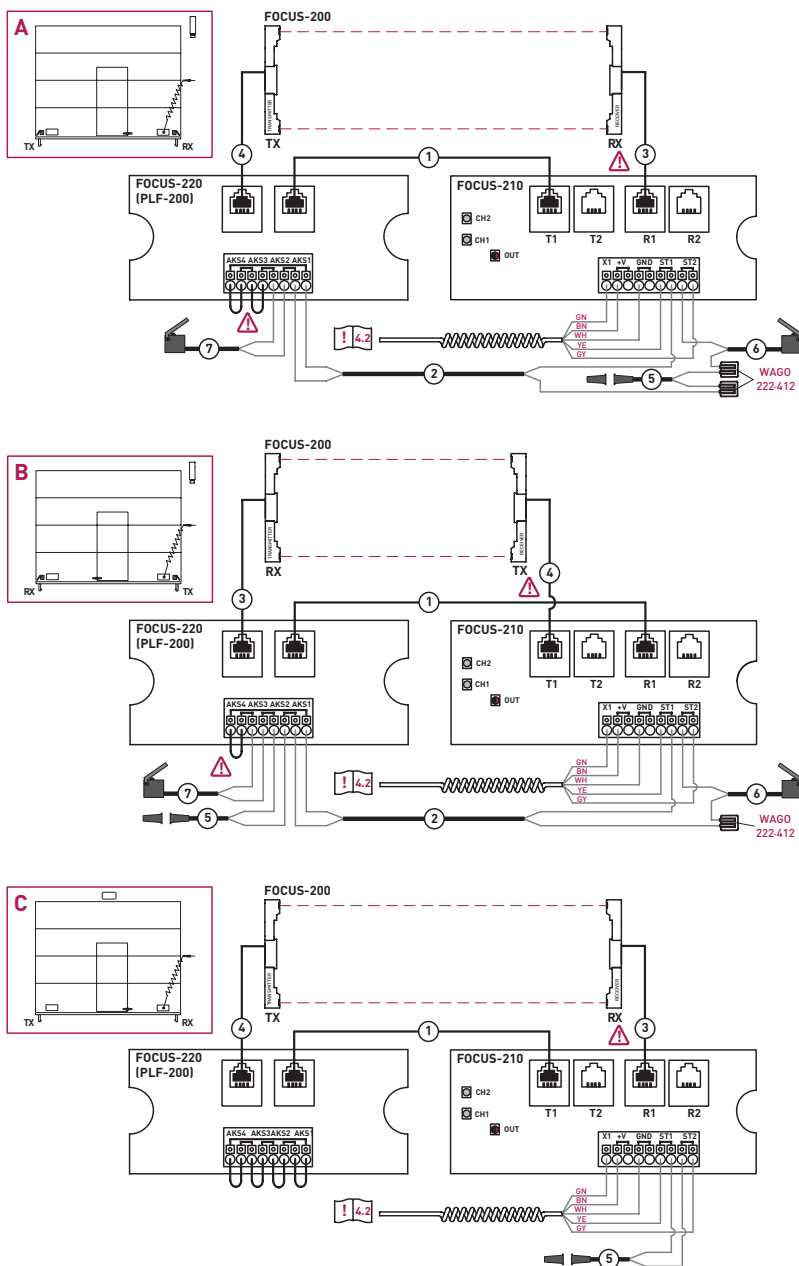
Рис. 3 — Примеры электрических подключений комплекта FOCUS-200KIT
